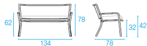
Āra atpūtas divāns Athena, tērauda rāmis Art. 3417 Cena 1367,00 EUR
