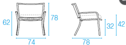
Āra atpūtas krēsls Athena, tērauda rāmis Art. 3416 Cena 767,00 EUR
